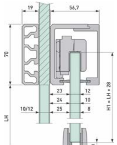
Montaje a fachada de vidrio Glass front installation
