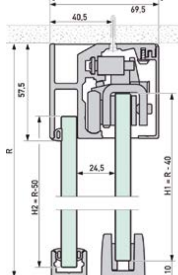
Montaje a techo con vidrio fijo Ceiling installation with fix glass
