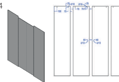
KIT MAMPARA 2 FIJOS-2 CORREDERAS 90° 8 mm ACERO AISI 304 1200 x 1200 mm VX5G SHOWER ROOM SET 2 SLIDING-2 FIX 8 mm STEEL AISI 304 1200 x 1200 mm VX5G
